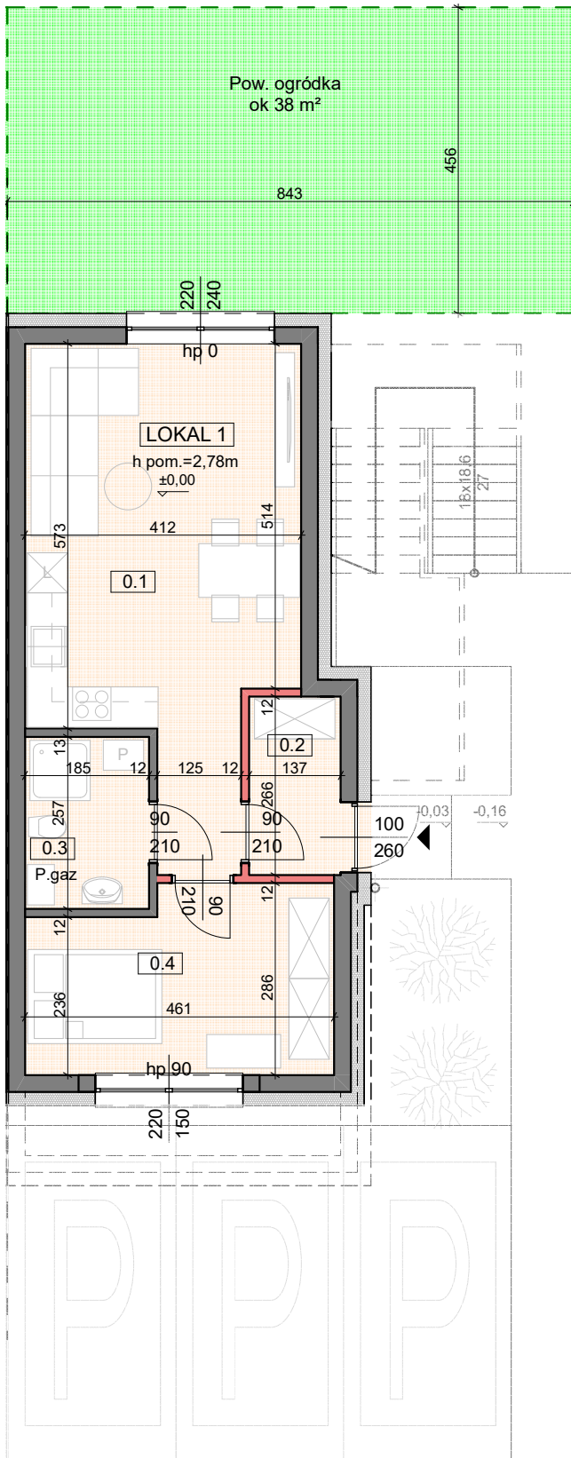
RZUT skala 1:100
